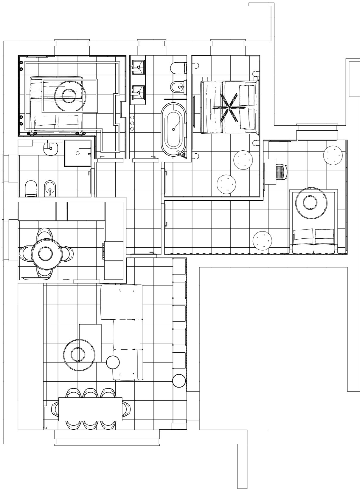
Planimetria Appartamento n.3
